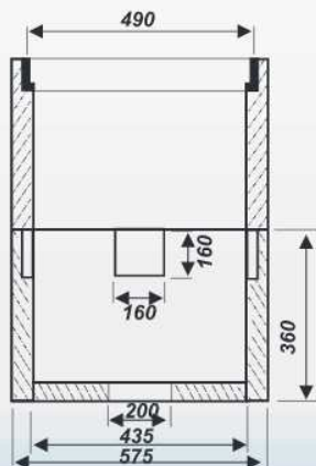
Przekrój poprzeczny
