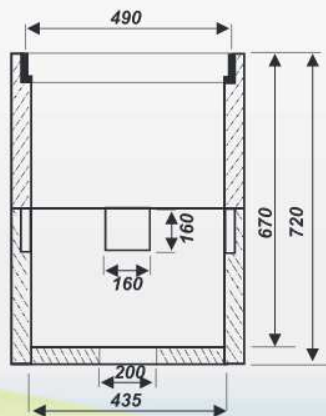
Przekrój podłużny
